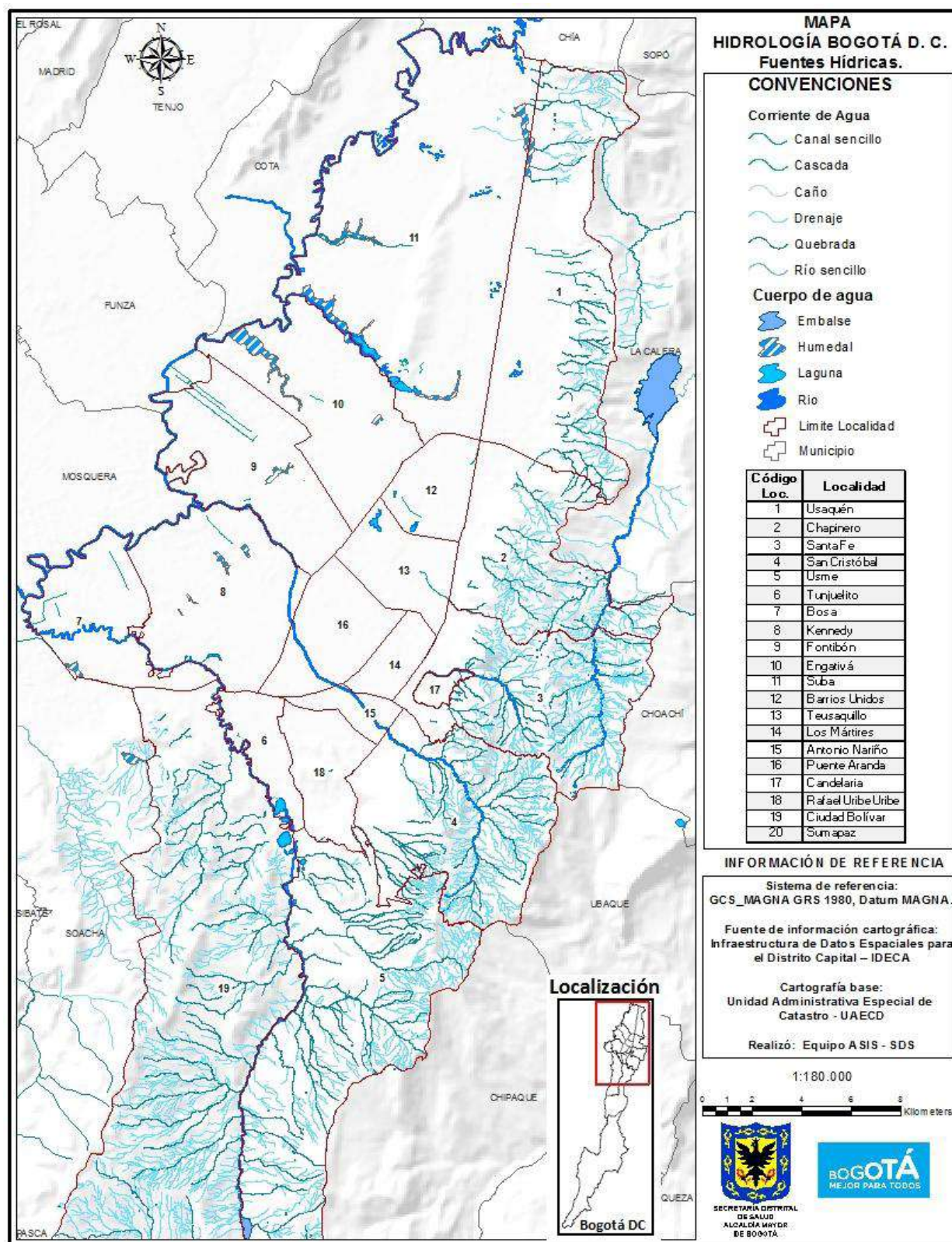
Mapa 4. Fuentes hídricas, Bogotá D. C., 2019
